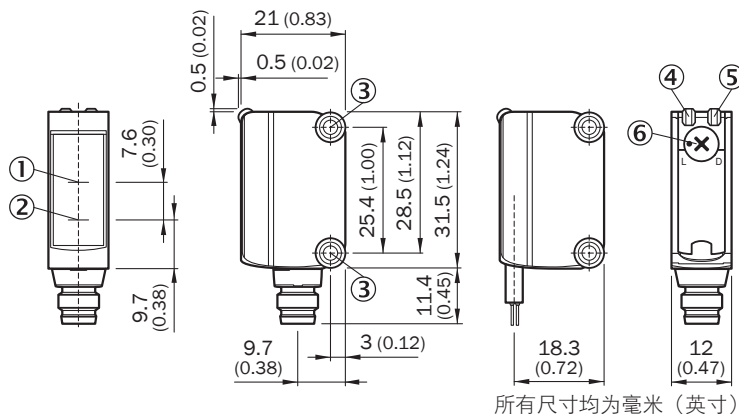
尺寸图
