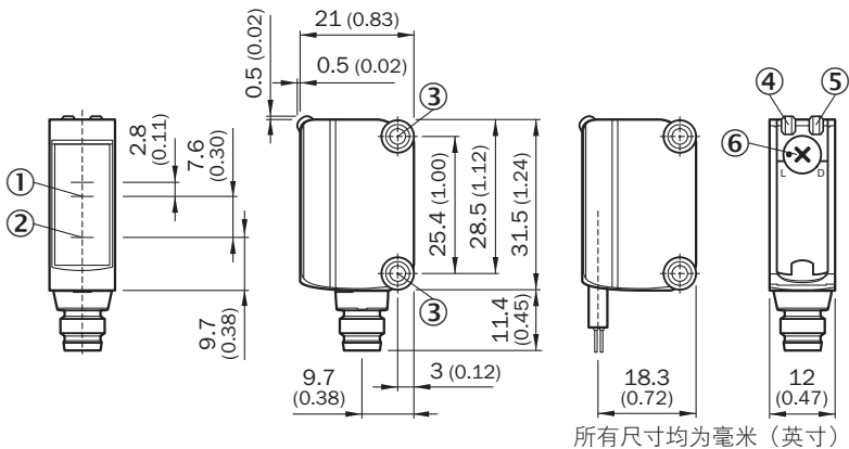
尺寸图
