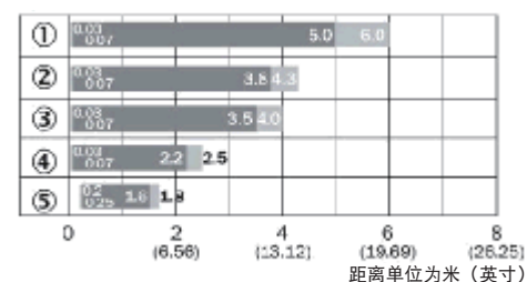
信号冗余
